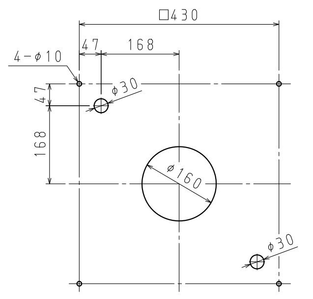
推奨据付寸法 (1:8)
